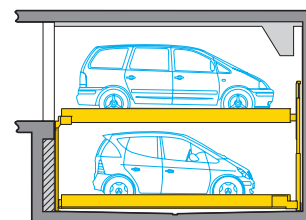
Schnittzeichnung | Section plan
